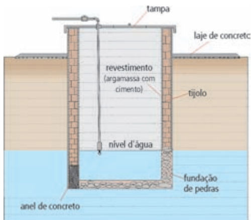
Esquema de um poço cacimba
